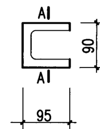
Q 90-3 压顶块
