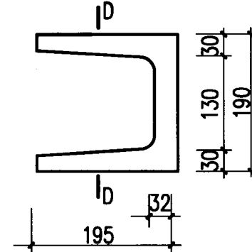
Q 190-3 过梁块
