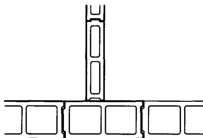
② 190厚与90厚墙 丁字交接奇数皮平面
