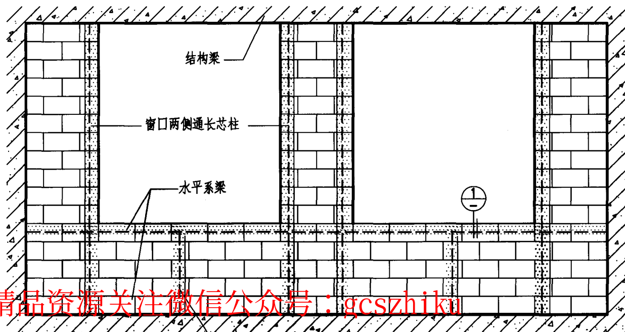
水泥聚苯颗粒 立面示例 保温砌块外墙
