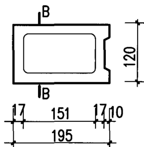
Q 120-2 半块
