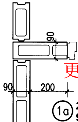
① 200宽 90厚墙垛
