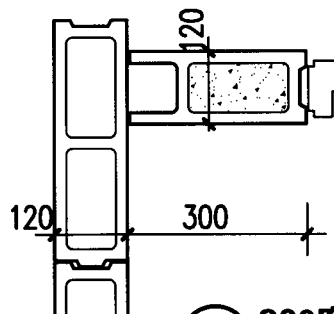
② 300宽 120厚墙垛
