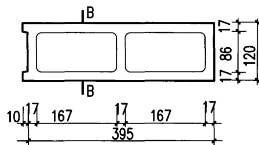
Q 120-1a 辅块(齐头块)
