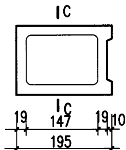
Q 140-2 半块
