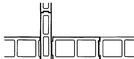
2a 190厚与90厚墙 丁字交接偶数皮平面
