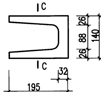
Q 140-3 过梁块
