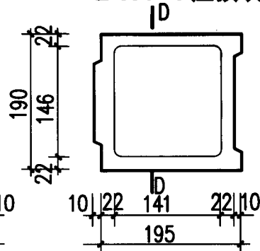
Q 190-2 半块
