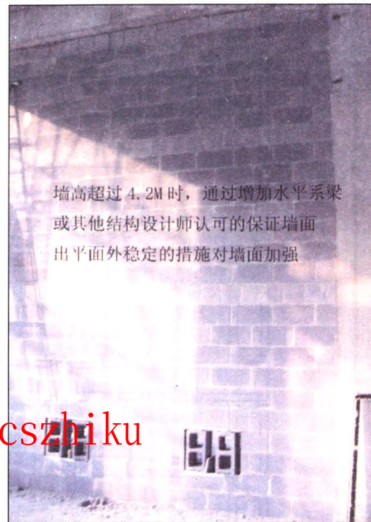
墙高 > 4.2m 时设两道水平系梁
