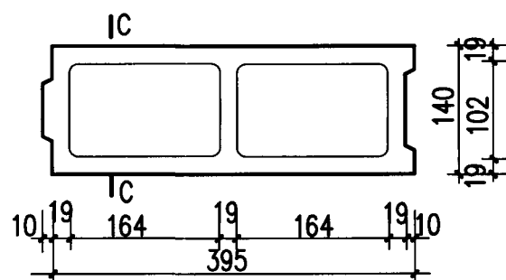
Q 140-1 主块
