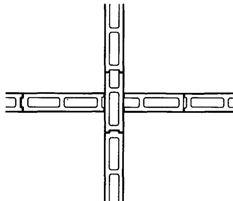
② 90厚墙十字交接 偶数皮平面
