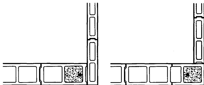
② 190厚与90厚墙转角处奇数皮平面
