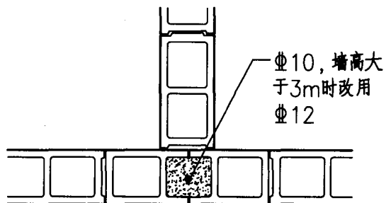
① 190厚墙丁字交接 奇数皮平面
