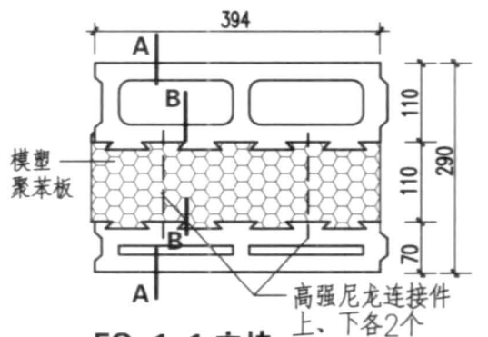
FQ-1-1 主块
