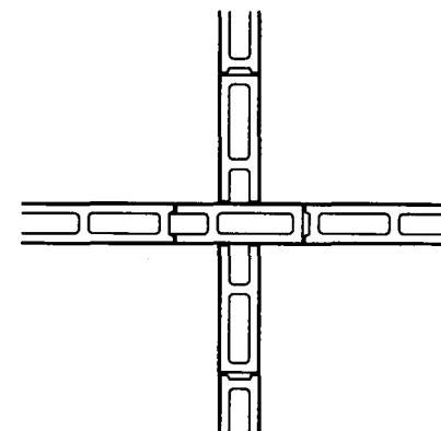
②a 90厚墙十字交接 奇数皮平面
