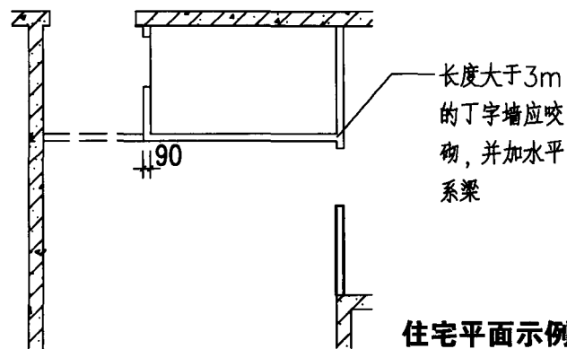
带门洞丁字墙
