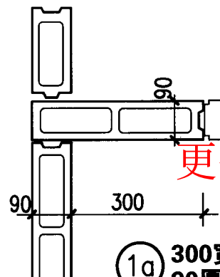
① 300宽 90厚墙垛
