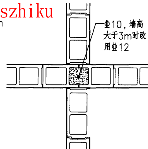
③a 190厚墙十字交接 偶数皮平面
