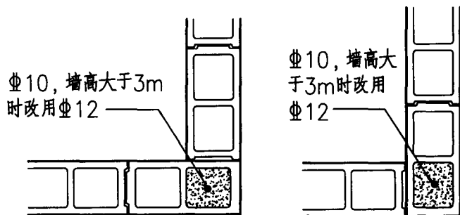
① 190厚墙转角部位奇数皮平面
