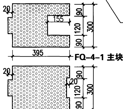
FQ-4-2 辅块
