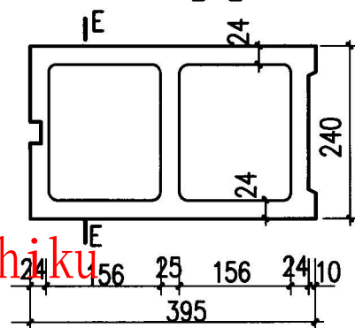
Q 240-1a 辅块 (洞边块)
