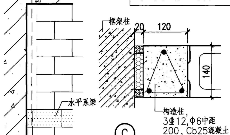
140厚砌块墙与 框架柱脱开的构造
