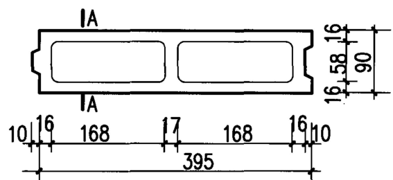
Q 90-1 主块
