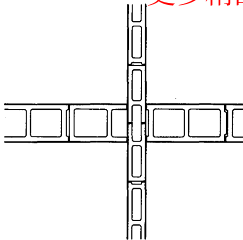
①a 190厚与90厚墙 十字交接偶数皮平面
