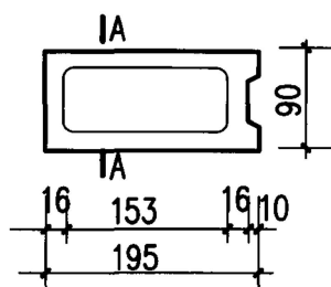
Q 90-2 半块
