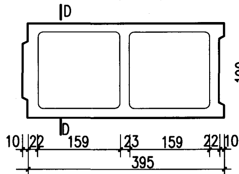
Q 190-1 主块
