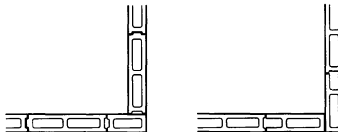
③ 90厚墙转角处奇数皮平面
