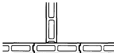
3a 90厚墙丁字交接 奇数皮平面
