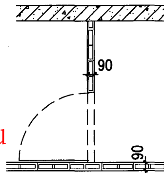
带门洞丁字墙
