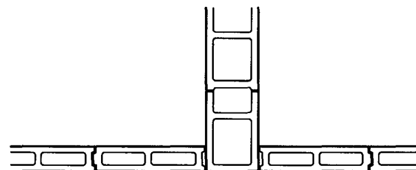
4a 90厚与190厚墙 丁字交接偶数皮平面
