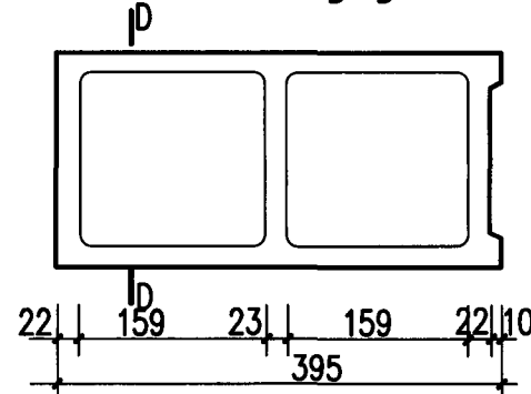
Q 190-1a 辅块 (齐头块)
