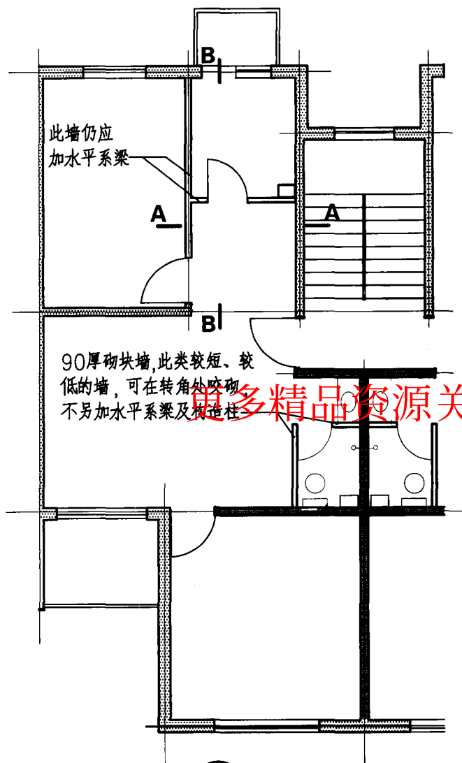
① 住宅平面示例
