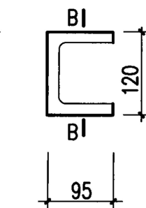
Q 120-3 压顶块
