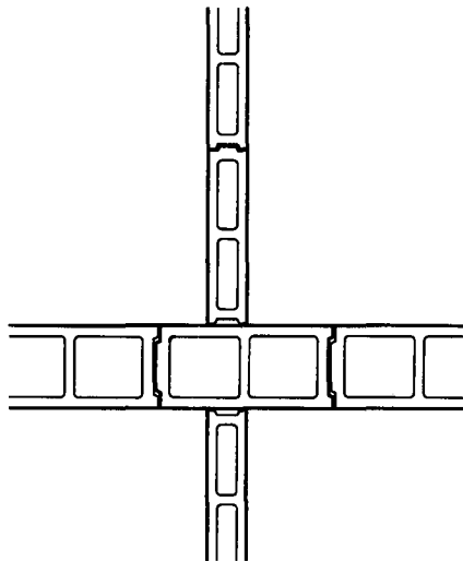
① 190厚与90厚墙 十字交接奇数皮平面
