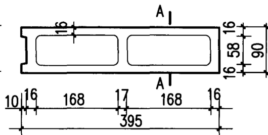
Q 90-1a 辅块(齐头块)
