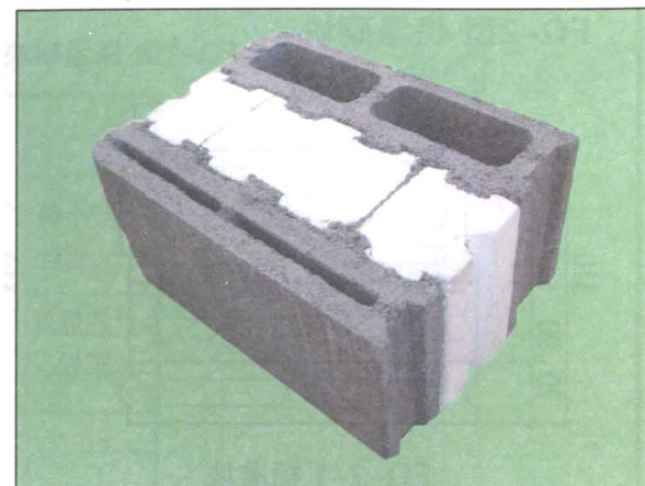
FQ-1 保温砌块 砌块检测传热系数为 0.32 \text{ W}/(\text{m}^2 \cdot \text{K})
