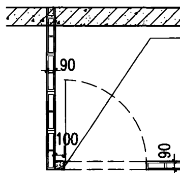
带门洞转角墙
