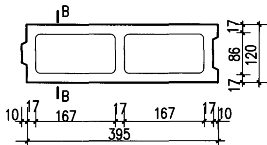
Q 120-1 主块
